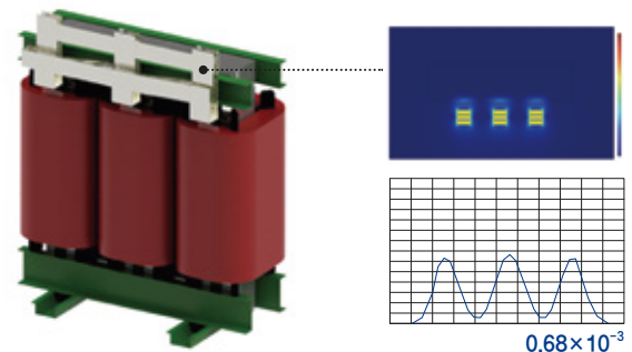
Hybrid 변압기
