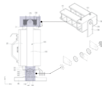
당사 마찰댐퍼
