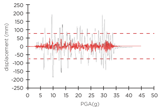
<규모 0.8g 가진 시 시간변위>
