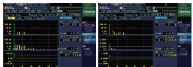
설치 전: 고효율 몰드 600 kVA
