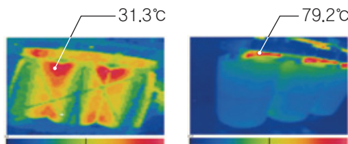
HV 권선
