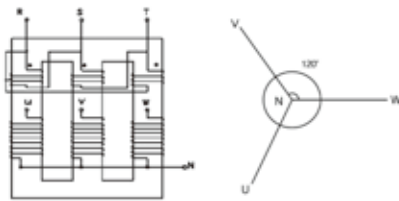
기존 변압기 Normal Winding
