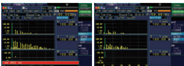
설치 전: 고효율 몰드 150 kVA
