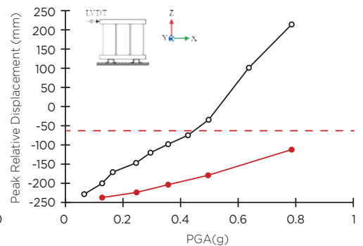
<PGA 대비 PRG>
