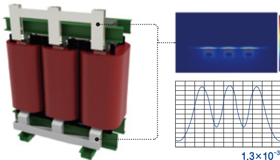
기존 변압기
